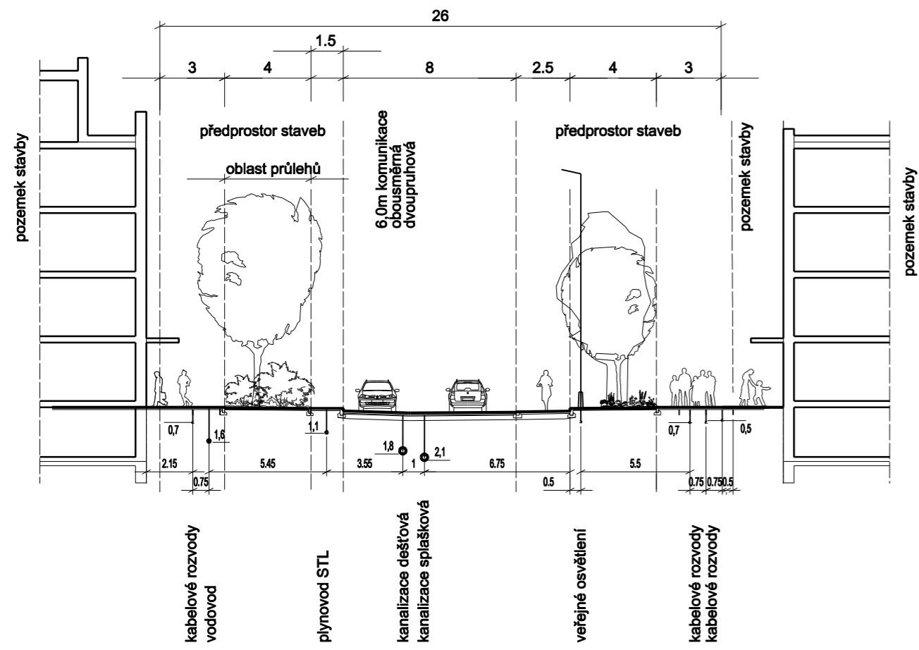
veřejné prostranství ulice (větev 1D průjezdná komunikace k pile) - řez 1-1
