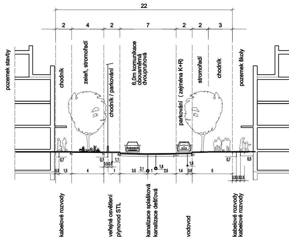
veřejné prostranství ulice (větev 2A u školy) - řez 2-2
