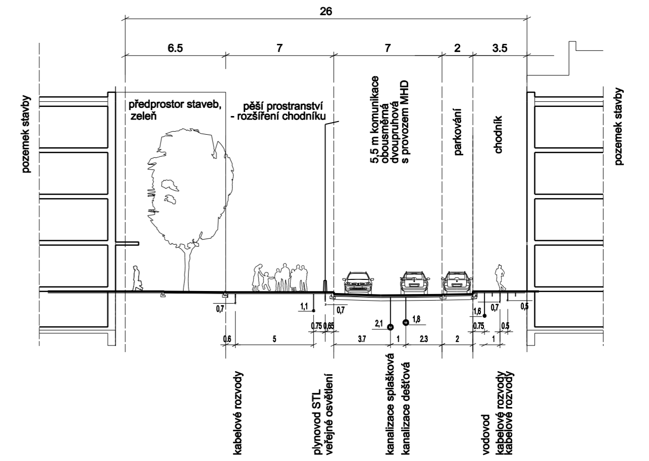
veřejné prostranství ulice (větev 4C obslužná komunikace k náměstí) - řez 4-4
