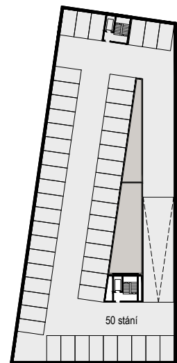
2.-3.PP
