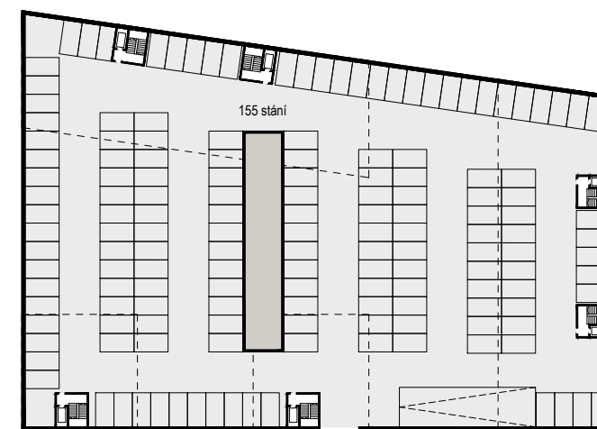
VJEZD GARÁŽE
