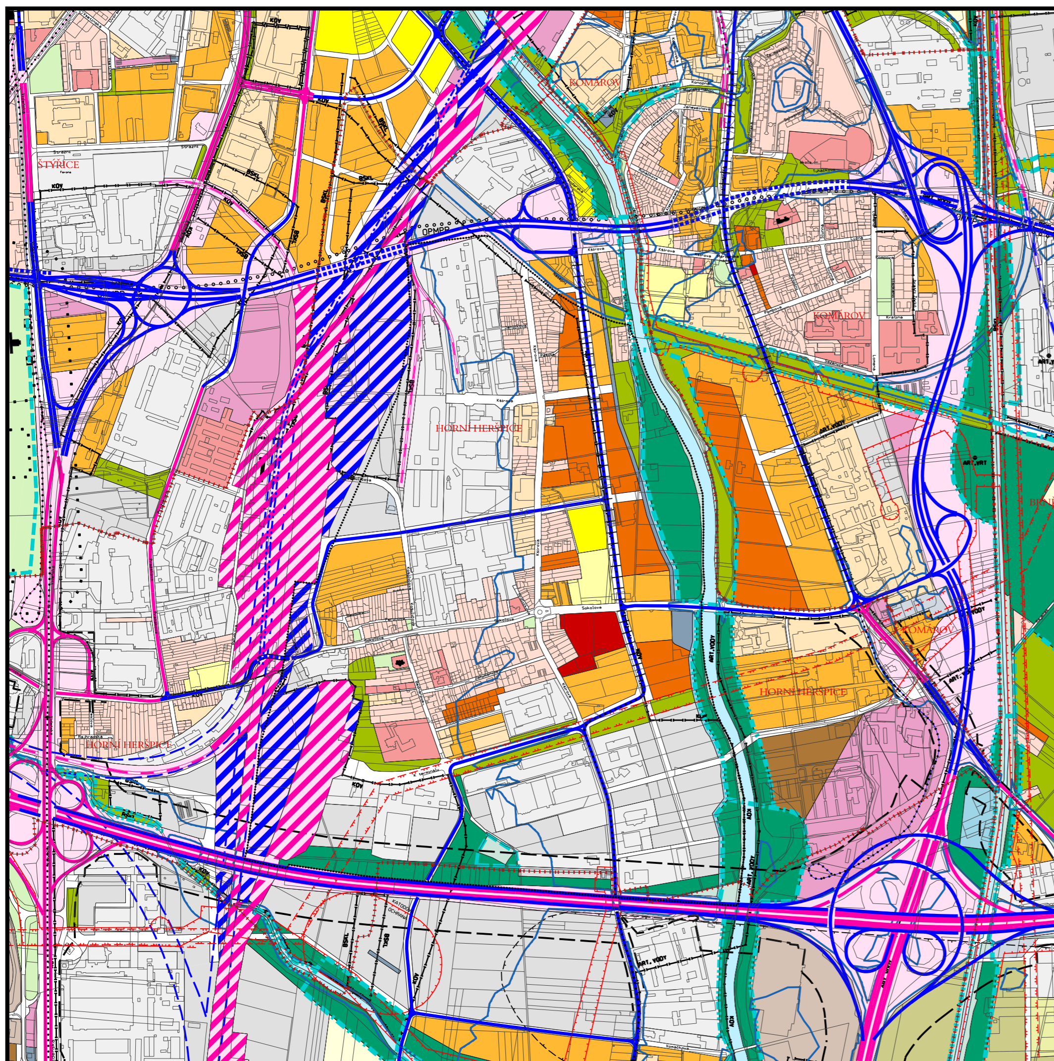
ŠIRŠÍ VZTAHY 1 : 10 000 - dle dohody z jednání 9.11.2005 (legenda dle ÚPmB) - bez napojení na D1 - s napojením na Bratislavskou radiálu v prodloužené Sokolově
