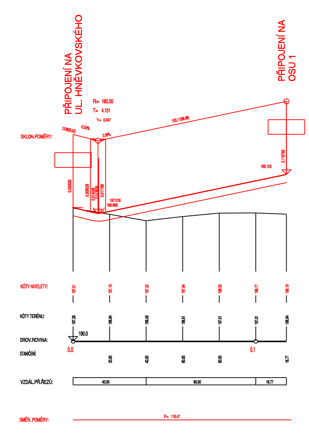
PODÉLNÝ PROFIL 1:1000/100 OSA 2 : UL. HNĚVKOVSKÉHO - OSA 1
