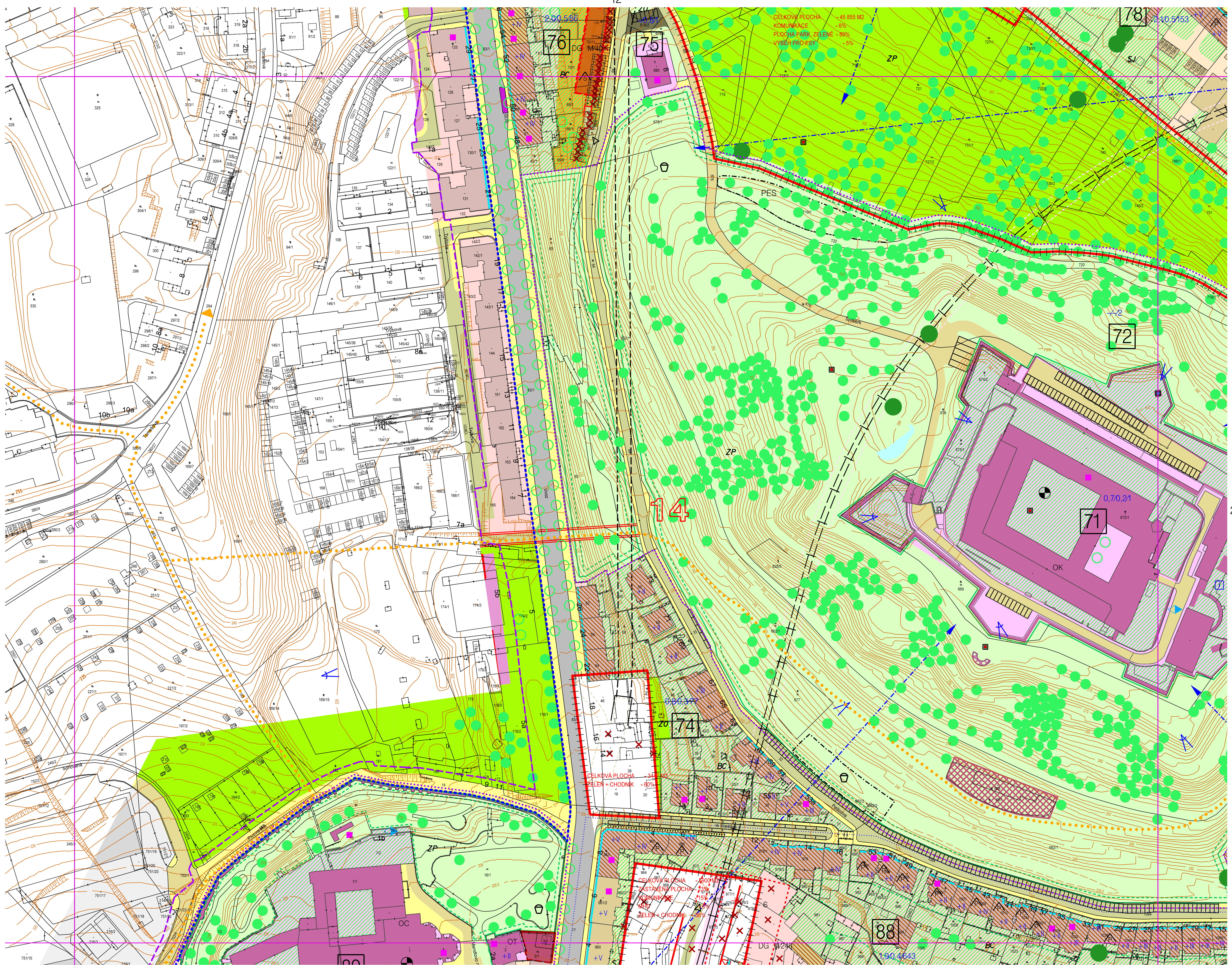
REGULAČNÍ PLÁN MPR BRNO, M 1 : 1000, BLOKY: 71, 72, 74, 75, 76, 78, 88, 89
